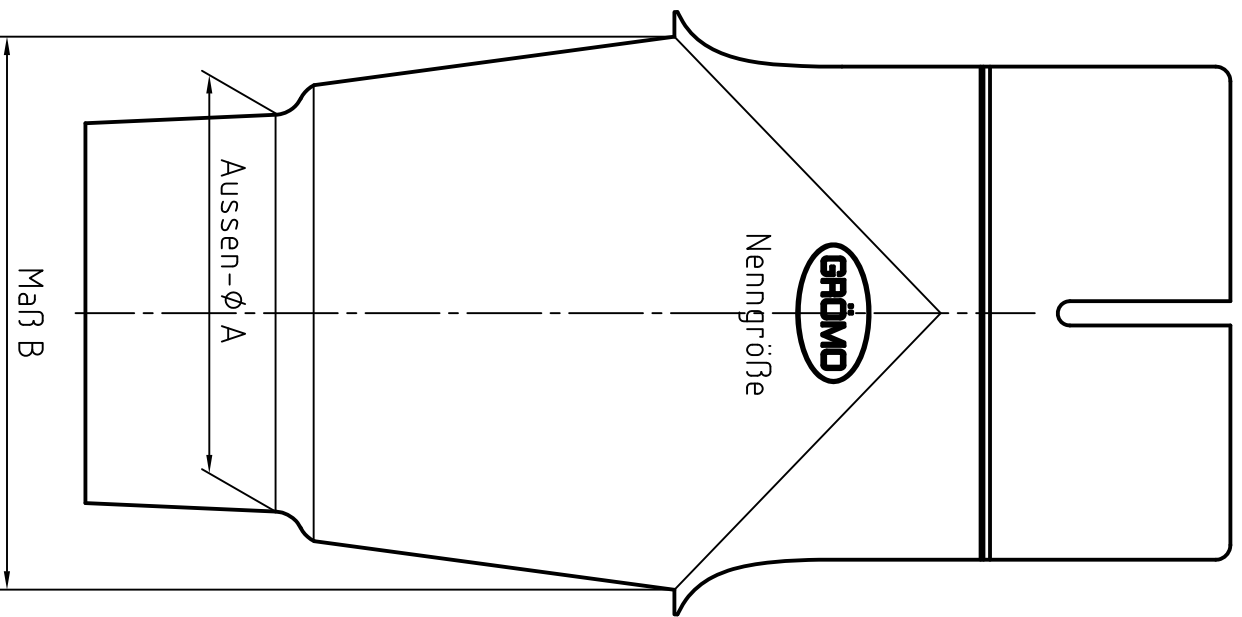
Vorderansicht
