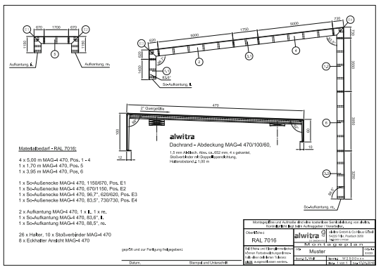
Beispiel CAD-Montageplan
