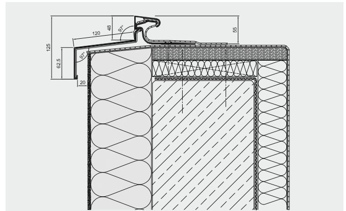
Montage über WDVS
