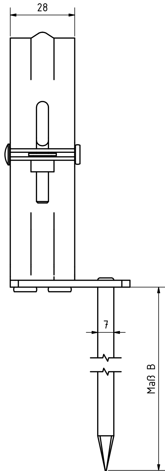
Seitenansicht
