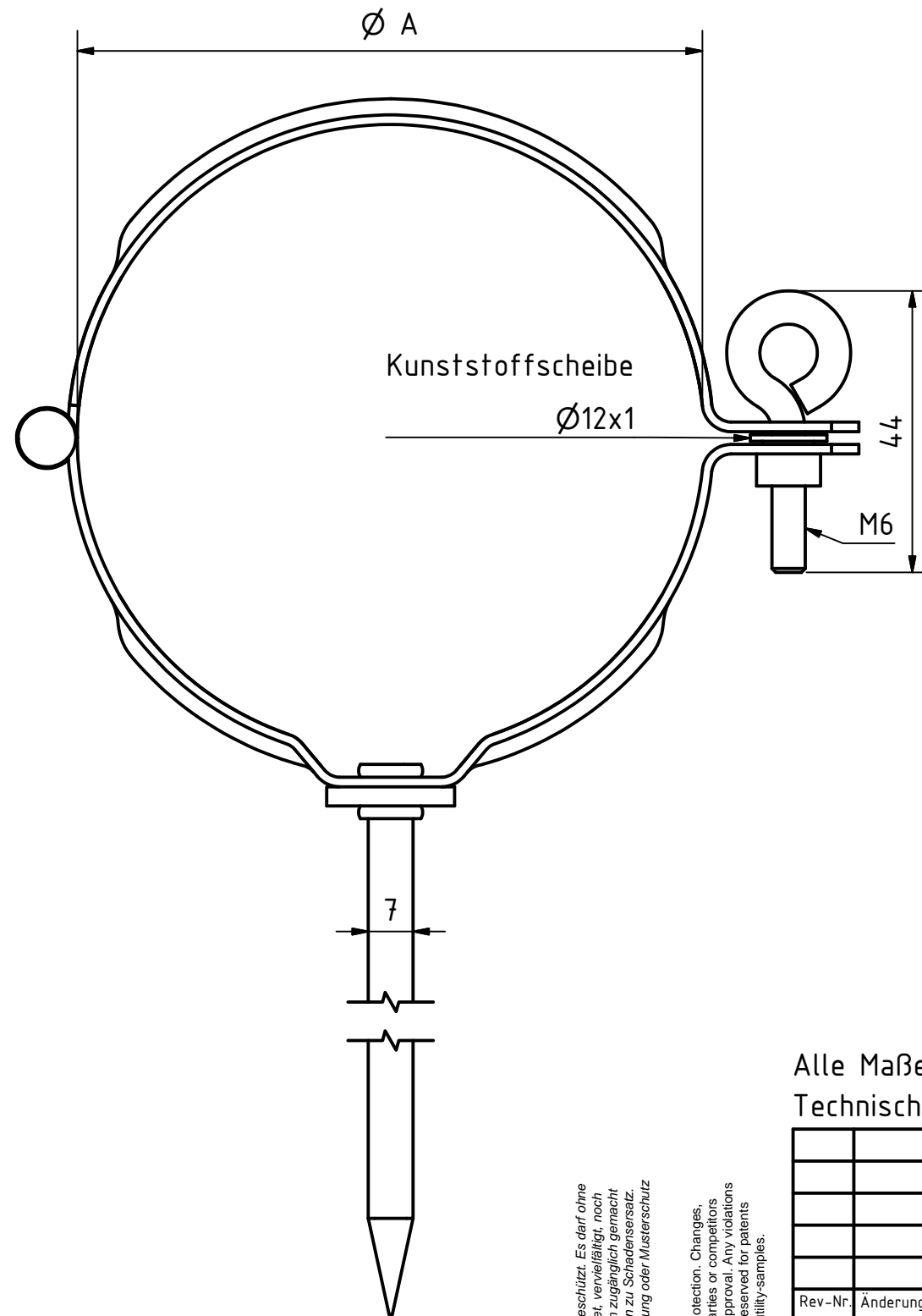
Draufsicht
